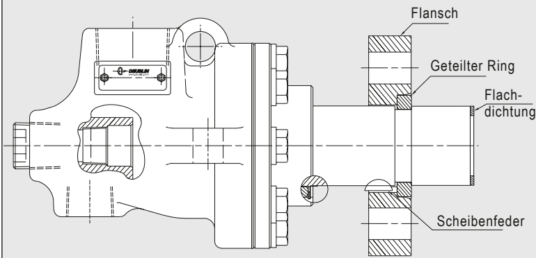
Flanschverbindung BC-54XXX-XX-30
