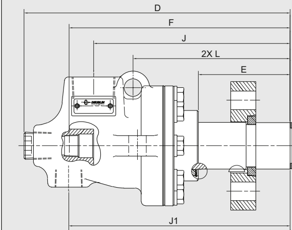
Flanschverbindung BC-54XXX-XX-30
