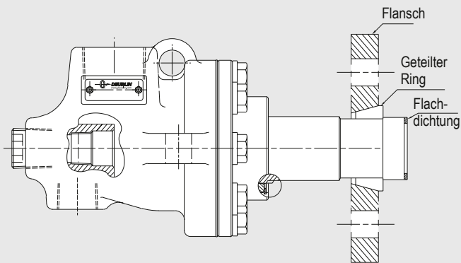
Losflansch Verbindung BC-54XXX-XX-32
