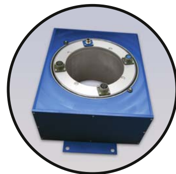
Schleifring für die industrielle Steuerung, Montage auf einer 165-mm-Welle
