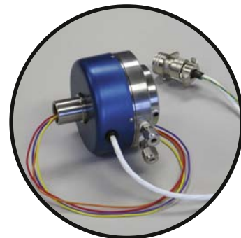
Kombination aus Schleifring und Drehdurchführung in einer integrierten Baugruppe
